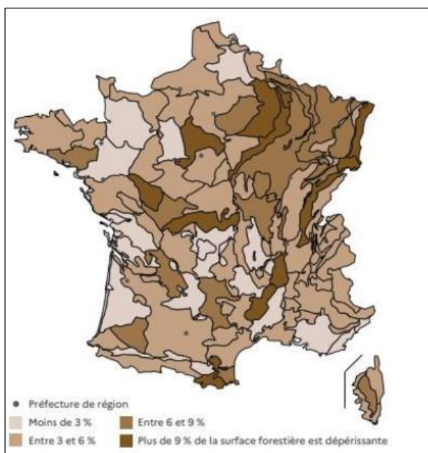
Figure 2 Taux de déperissement apparent des peuplements forestiers par sylvoécocorégion, campagnes d'inventaire forestier 2018-2022. Seuil individuel de l'arbre \geq 50 % de branche morte ; seuil de peuplement \geq 20 % des arbres déperissants. Source : IGN.
