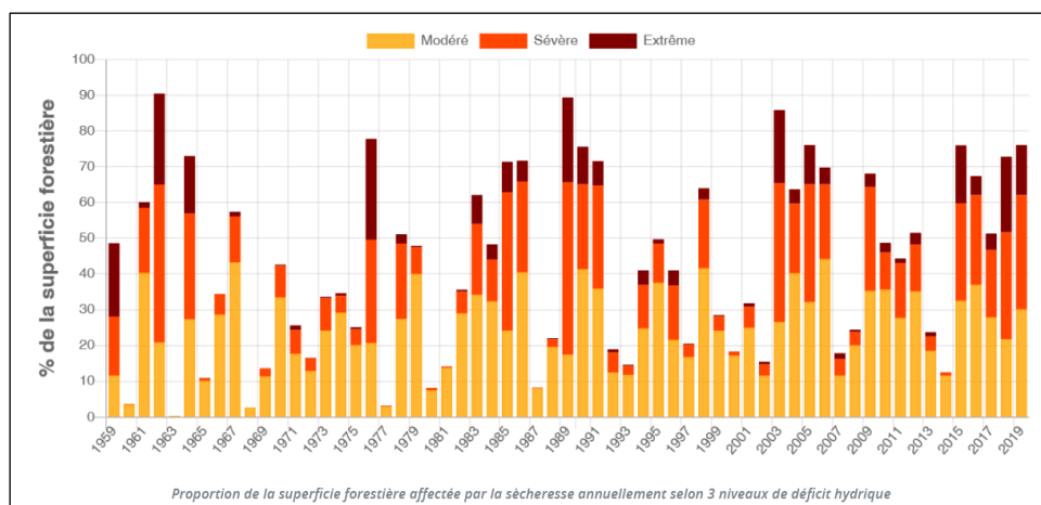
Figure 4 Proportion de la superficie de la forêt française affectée par la sécheresse (tous peuplements). Source : IGN
