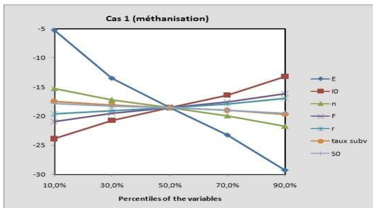
Figure 31: Diagramme représentant pour chaque paramètre son impact, selon sa position dans les différents déciles (en abscisse), sur le coût complet calculé (en ordonnée) – Source: calcul de la mission
