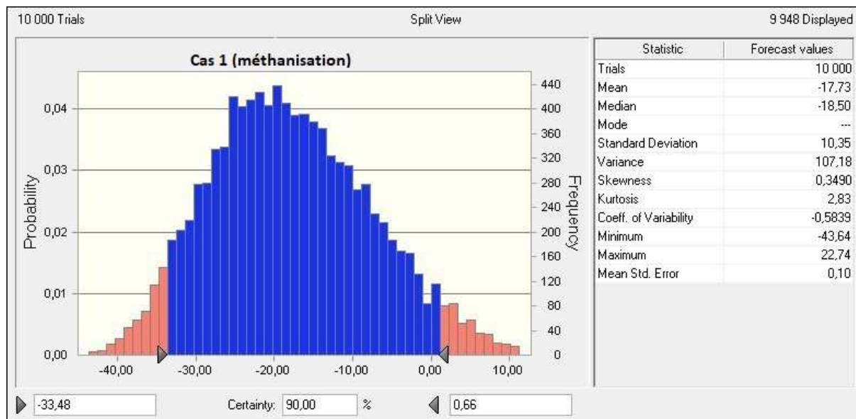
Figure 30: Histogramme de la distribution des valeurs de coût complet de l'énergie (en abscisse, €/Mwh) ; pour chaque valeur de coût en abscisse, l'ordonnée correspond à sa densité de probabilité; les valeurs en bleu correspondent à une probabilité cumulée de 90 % - Source : calcul de la mission
