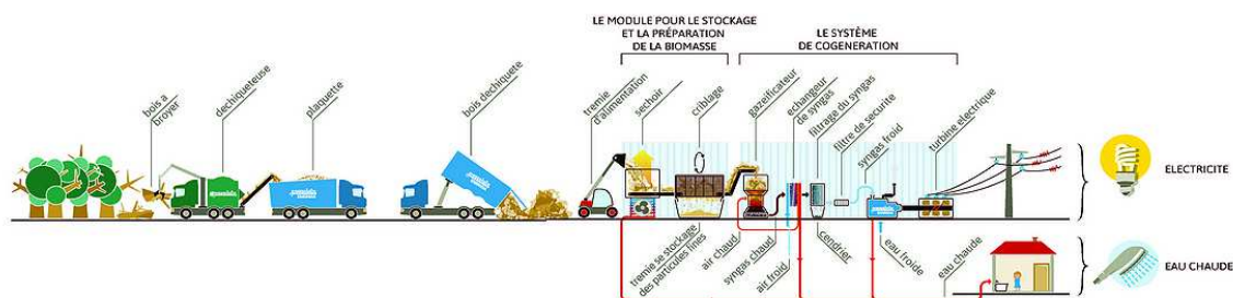
Figure 16: Schéma de la cogénération, Source : www.picbleu.fr
