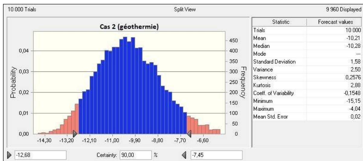
Figure 32: Histogramme de la distribution des valeurs de coût complet de l'énergie (en abscisse, €/Mwh) dans un cas d'installation géothermique; pour chaque valeur de coût en abscisse, l'ordonnée correspond à sa densité de probabilité; les valeurs en bleu correspondent à une probabilité cumulée de 90 % - Source : calcul de la mission
