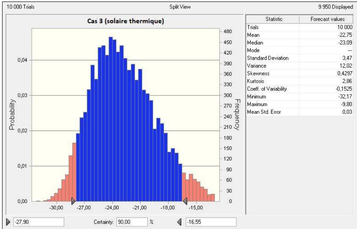
Figure 34: Histogramme de la distribution des valeurs de coût complet de l'énergie (en abscisse, €/Mwh) dans un cas d'installation solaire thermique; pour chaque valeur de coût en abscisse, l'ordonnée correspond à sa densité de probabilité; les valeurs en bleu correspondent à une probabilité cumulée de 90 % – Source, calcul de la mission
