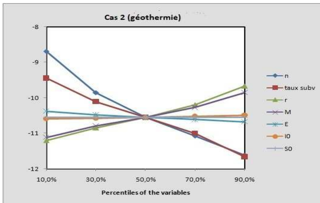
Figure 33: Diagramme représentant pour chaque paramètre son impact, selon sa position dans les différents déciles (en abscisse), sur le coût complet calculé (en ordonnée) – Source : calcul de la mission
