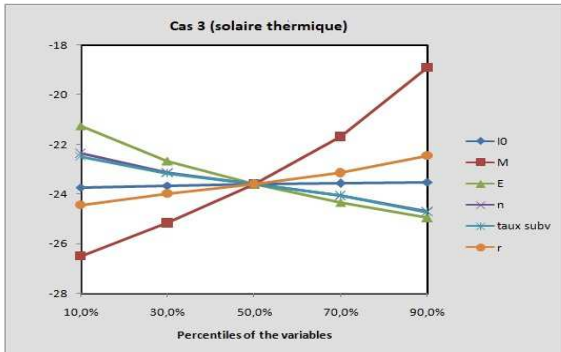
Figure 35: Diagramme représentant pour chaque paramètre son impact, selon sa position dans les différents déciles (en abscisse), sur le coût complet calculé (en ordonnée) – Source : calcul de la mission
