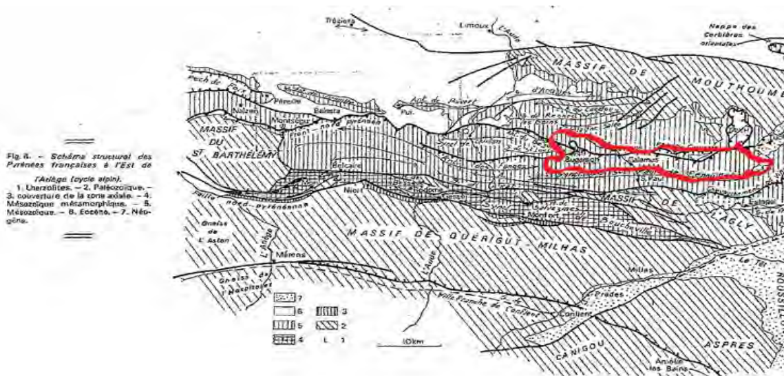
Fig 1 : Géologie du sud des Hautes- Corbières (JAFFRIEZO M., 1977)
