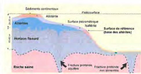
Figure 3 : Modèle conceptuel des altérités superposées en domaine granitique (B. Wynn 2004) 12
